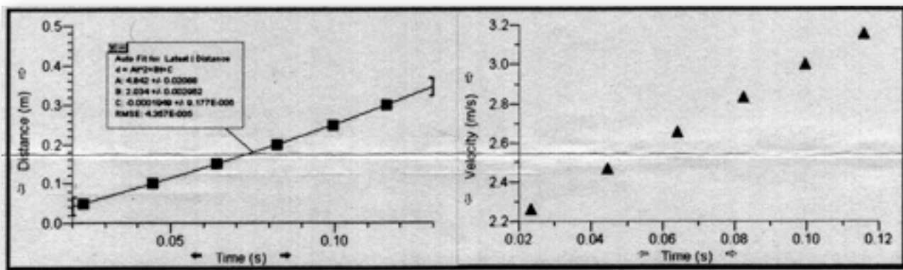
Príklady grafov pádu pravítka cez fotobránu (závislosti dráhy a rýchlosti od času)
